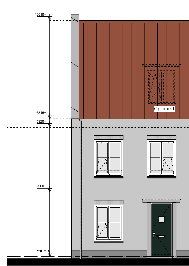
VOORGEVEL bnr 14
