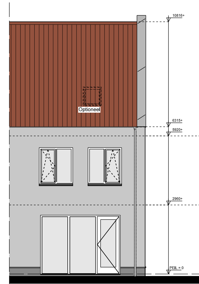
ACHTERGEVEL bnr 14
